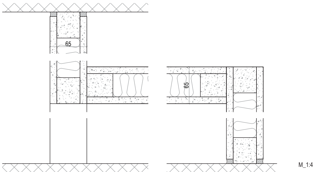
Cloison de séparation (coupe verticale)
