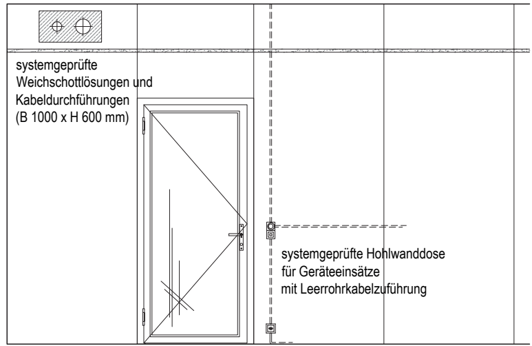
Option d'exécution passages électriques (élévation)
