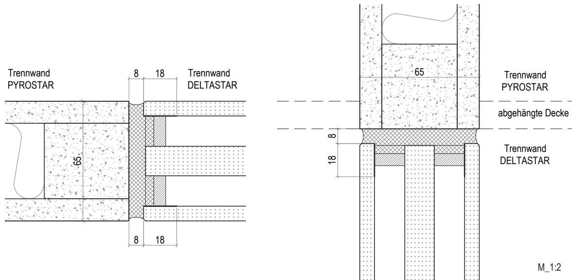
Paroi de séparation avec raccord paroi vitrée DELTASTAR (coupe horizontale/verticale)
