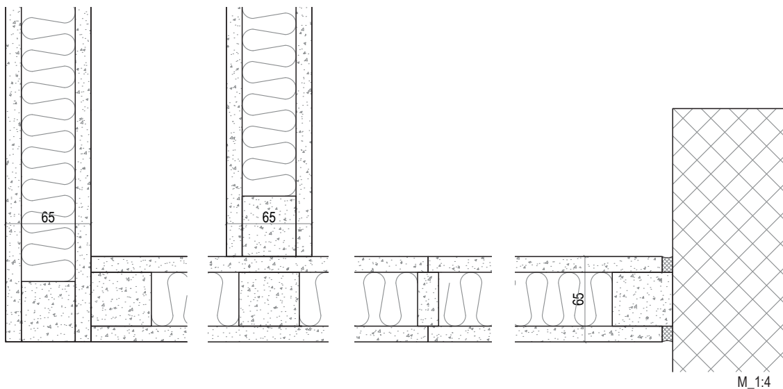
Détail d'angle et de raccord (coupe horizontale)
