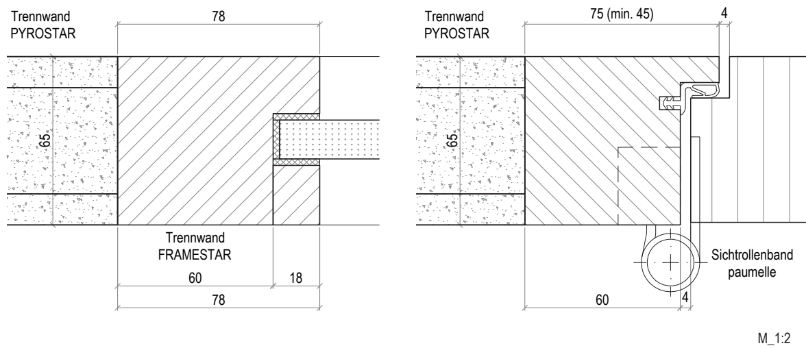
Paroi de séparation avec raccord à la paroi vitrée FRAMESTAR et à la porte en cadre bloc (coupe horizontale)
