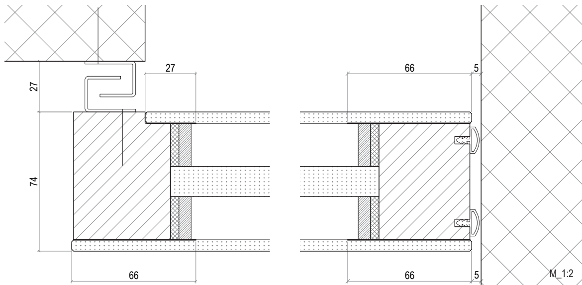
Exécution 1 vantail (coupe horizontale)
