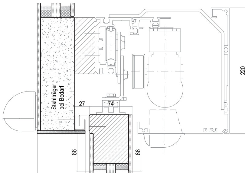
Raccord de la porte en verre DELTASTAR, détail de raccord au plafond (coupe verticale)
